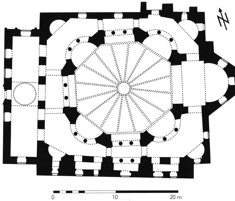
Afbeelding 8. Sergius en Bacchuskerk, Istanbul, plattegrond. Uit: N. Asutay-Effenberger en A. Effenberger, Byzanz. Weltreich der Kunst (München 2017) afb. 30.
