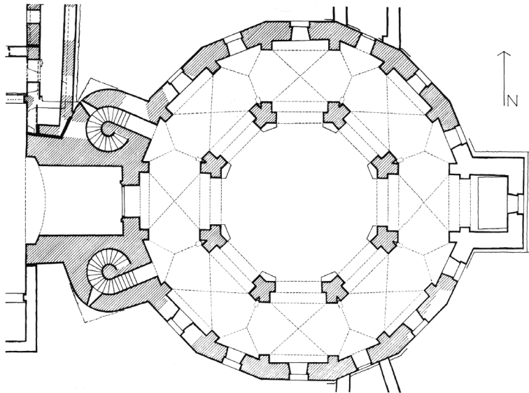
Afbeelding 10. Paltskapel, Aken, plattegrond. Centrum voor Kunsthistorische Documentatie, Radboud Universiteit.
