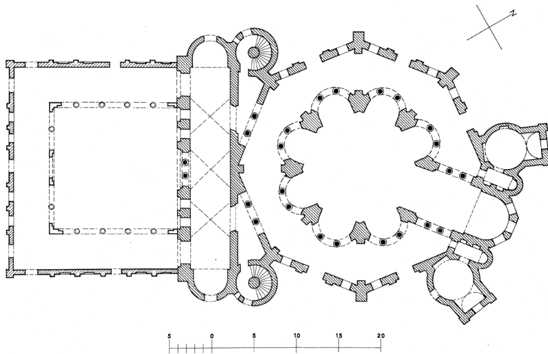
Afbeelding 6. San Vitale, Ravenna, plattegrond . Uit: F.W. Deichmann, Ravenna. Hauptstadt des spätantiken Abendlandes II, 2 (Wiesbaden 1976) Plan 37.
